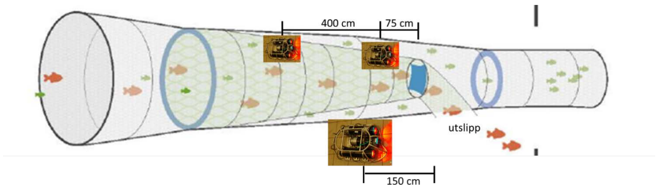
Figur 4: Plassering av GoPro Hero 4-kameraer på Excluder. To kameraer ble plassert i innerrøret og et i utslippet.
