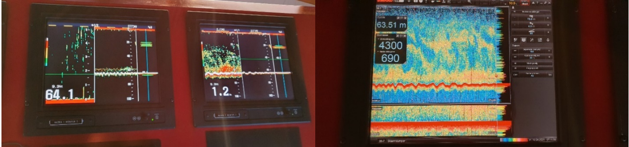
Figur 3: Ekkogrammer på Engelsk Klondyke nord, 10.04.2021 kl. 07:00 CET. Til venstre er 50 kHz og 200 kHz ekkogrammer. Til høyre er 38 kHz ekkogram.
